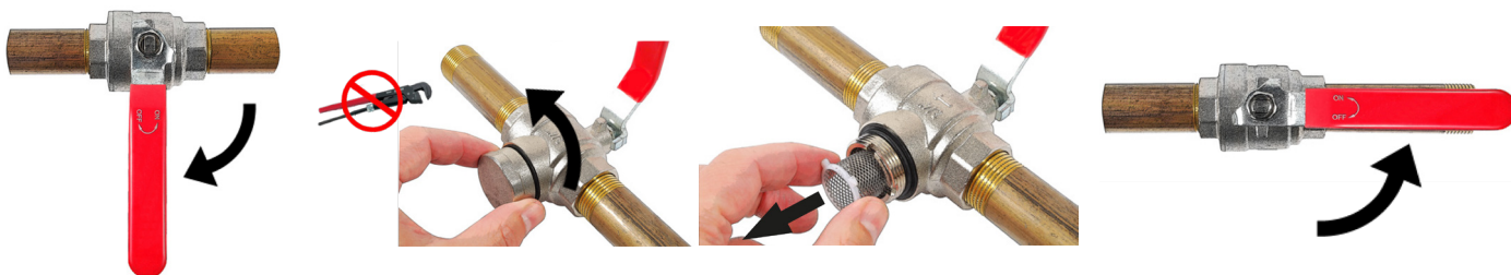
Obr. 6 - uzavření kohoutu
