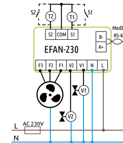
b) 4-toruline kliimakonvektor (kütmine ja jahutamine) või pörandaküte ja kliimakonvektor jahutamiseks
