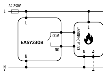
a) Ühendusskeem gaasikatlale
