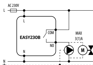
b) Ühendusskeem pumbale / ajamile
