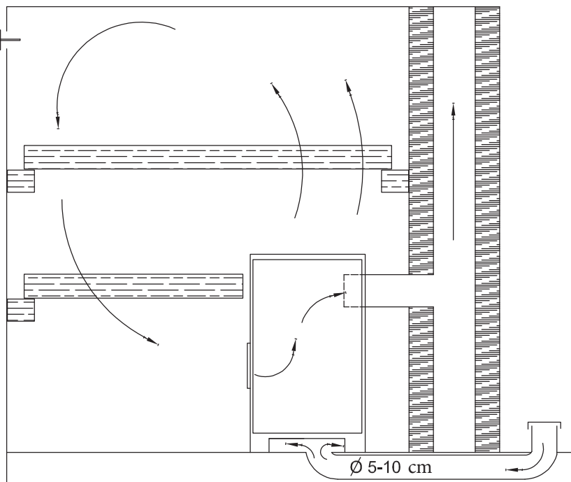
Joonis 1. Loomulik ventilatsioon Рисунок 1. Естественная вентиляция
